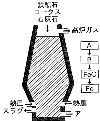
図 鉄の製錬
